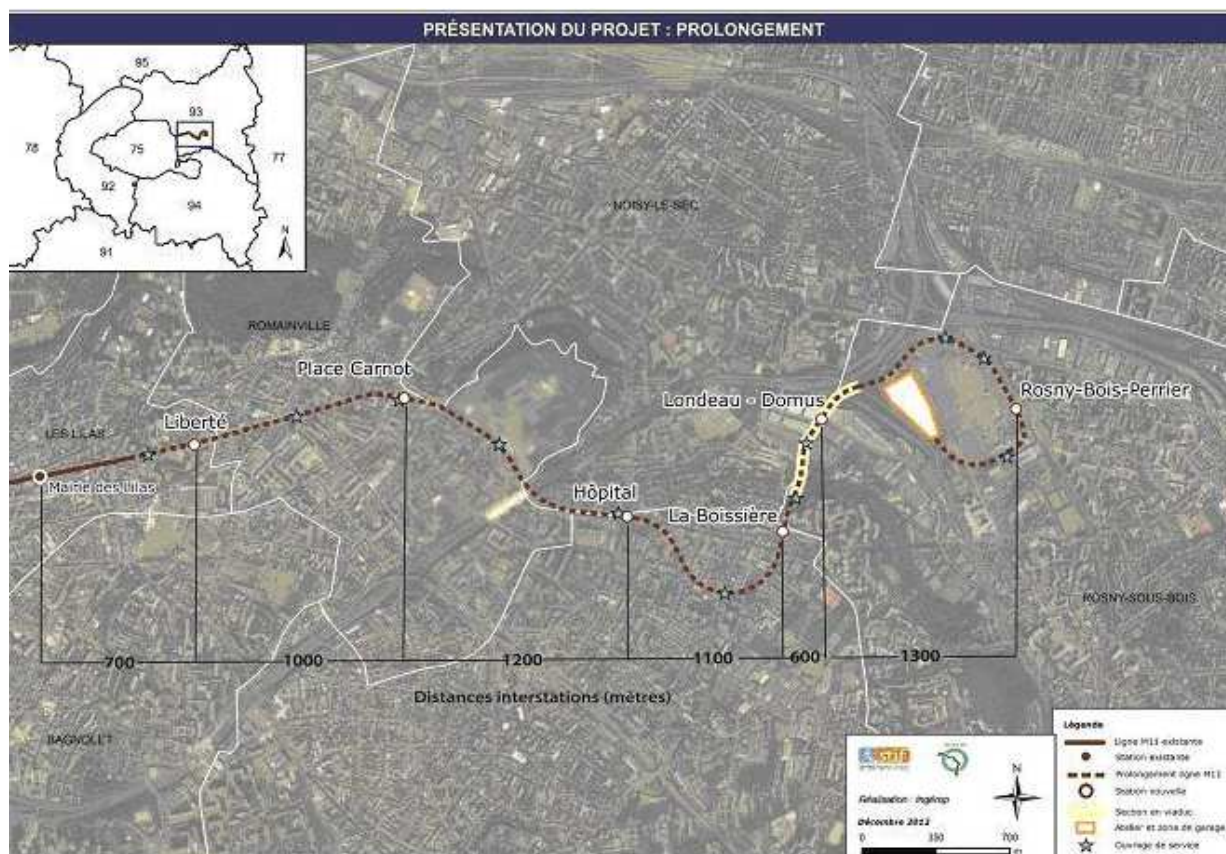
Figure 2 : Tracé du prolongement et localisation des futures stations de la ligne 11 (source: résumé non technique, pièce G, Chapitre II)
