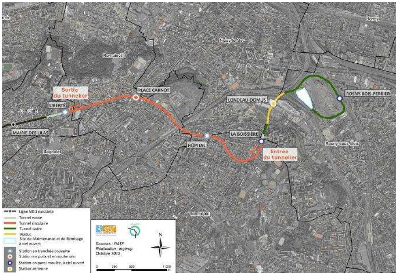
Figure 3 : méthodes de construction utilisées pour le prolongement de la ligne 11 (source : dossier d'enquête publique, pièce E, chapitre II)
