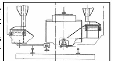
Éta bli avec tête de soudage (coupe) en place pour la 2 ème soudure et dispositif de refroidissement de la première soudure
