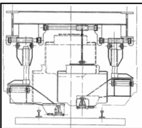
Éta bli avec tête de soudage (coupe) en place pour la deuxième soudure
